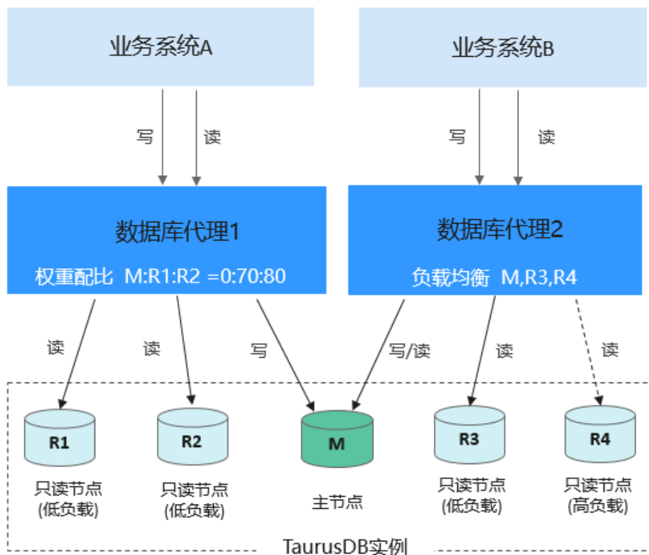
图 12-15 路由模式工作原理
